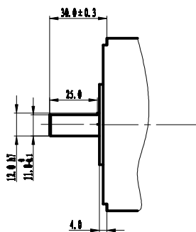
铣扁型 (GB) Milling flat
