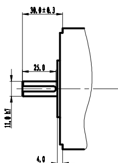
键槽型 (GA) Type keyway
