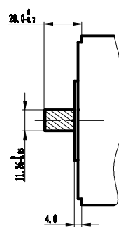
斜齿型 (GD) Helical tooth
