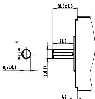
键槽型 (GA) Type keyway
