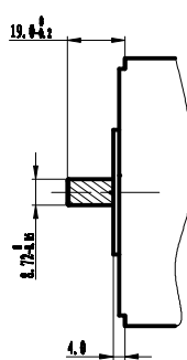
斜齿型 (GC) Helical tooth
