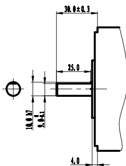
铣扁型 (GB) Milling flat
