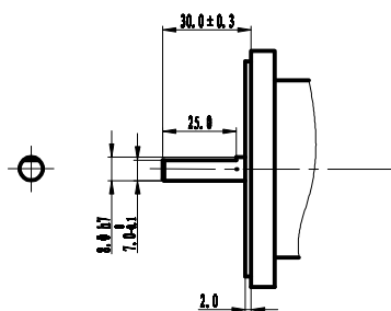
铣扁型 (GB) Milling flat
