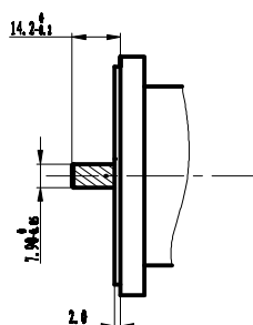
斜齿型 (GN) Helical tooth
