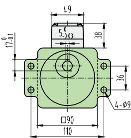
带耳减速箱
